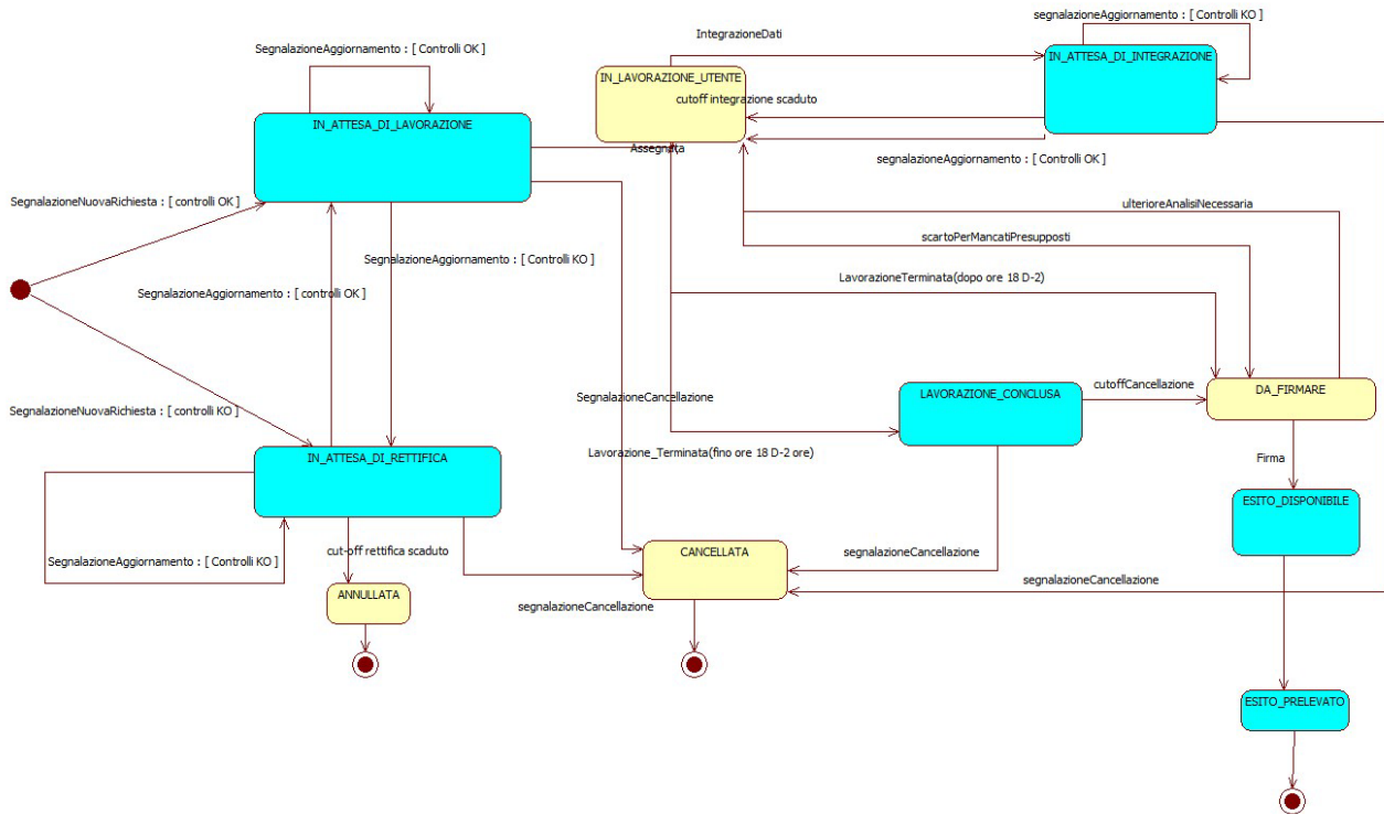
Figura 3 – Diagramma degli stati della richiesta di protesta
