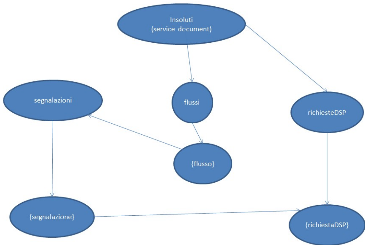
Figura 32 – Grafico dell'interfaccia REST dell'applicazione Insoluti
