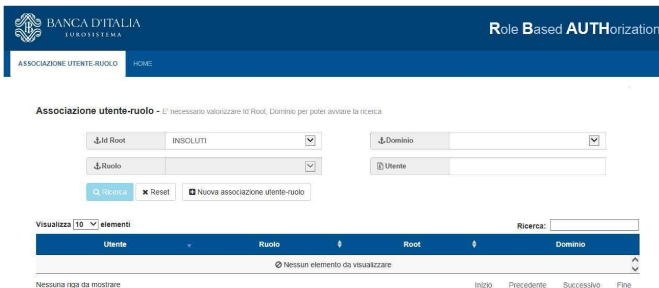
Figura 28 – Associazione utente-ruolo: selezione applicazione
