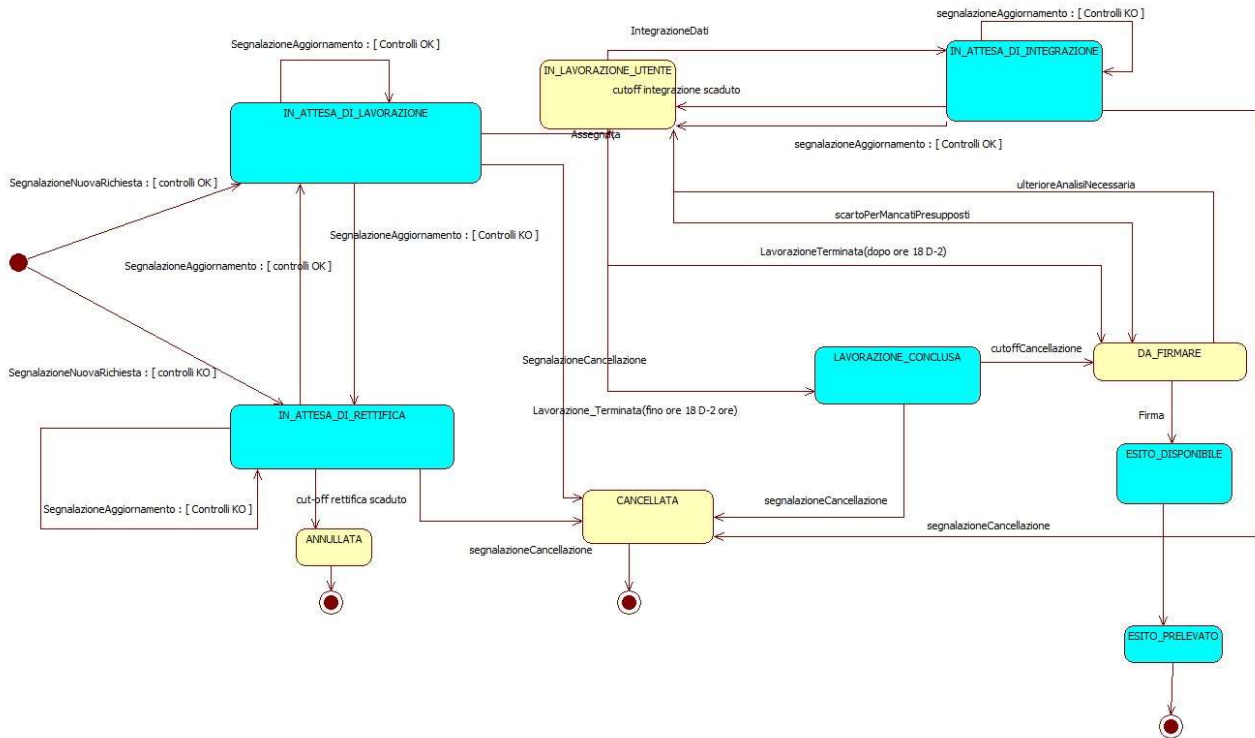
Figura 3 – Diagramma degli stati della richiesta di protesto
