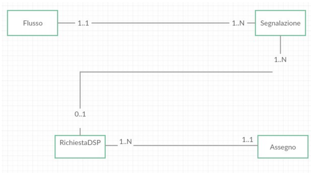
Figura 2 – Modellazione entità A2A
